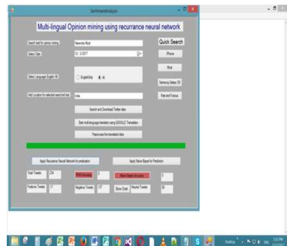
Fig. 10. Apply RNN
